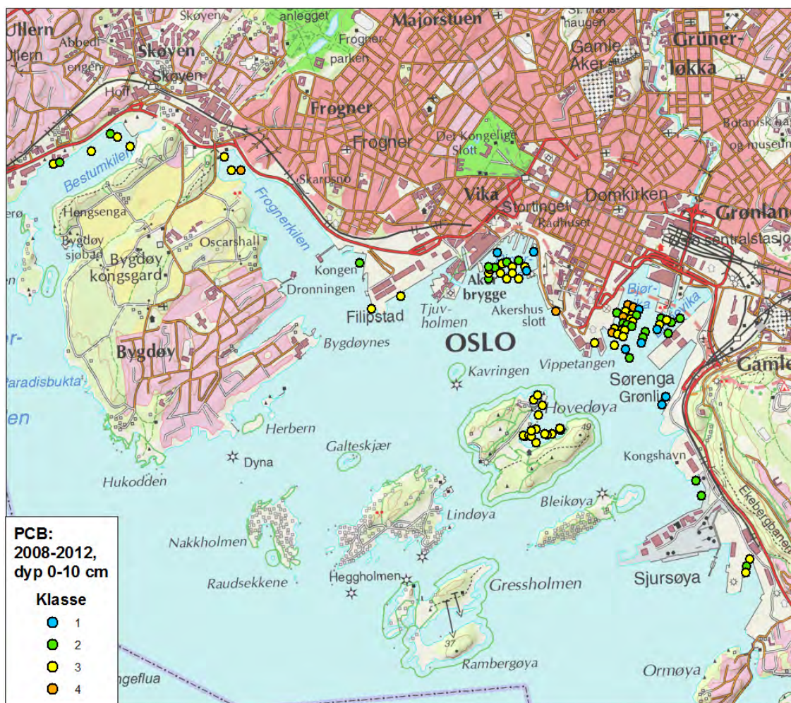
Figur 77. Resultater av klassifisering av miljøtilstand basert på Sum PCB (summen av konsentrasjonen av 7 ulike PCB kongenerer, dvs. kongenerene 28, 52, 101, 118, 138, 153 og 180) i de øverste 0-10 cm av sedimentet i Indre Oslofjord, prøver tatt i perioden 2008-2012. Klassifiseringen er gjort i henhold til klassegrensene oppgitt i utkast til TA 3001/2012. Fargekodene brukt for de enkelte tilstandsklasser er vist i figuren.
