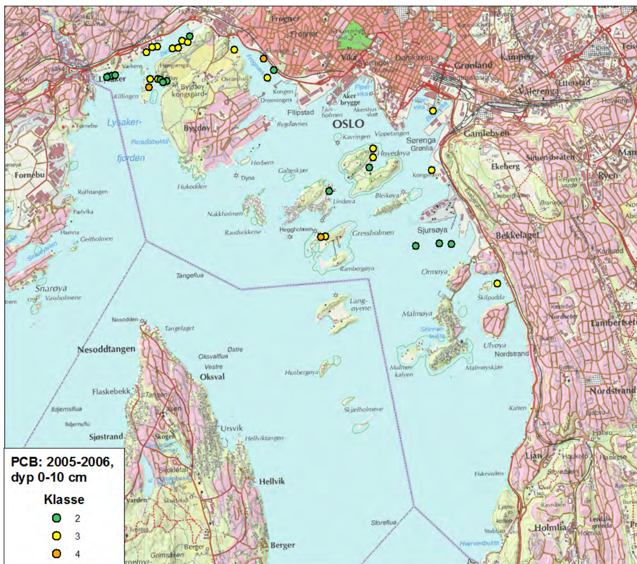
Figur 71. Resultater av klassifisering av miljøtilstand basert på Sum PCB (summen av konsentrasjonen av 7 ulike PCB kongenerer, dvs. kongenerene 28, 52, 101, 118, 138, 153 og 180) i de øverste 0-10 cm av sedimentet i Indre Oslofjord. Klassifiseringen er gjort i henhold til klassegrensene oppgitt i utkast til TA 3001/2012. Fargekodene brukt for de enkelte tilstandsklasser er vist i figuren.
