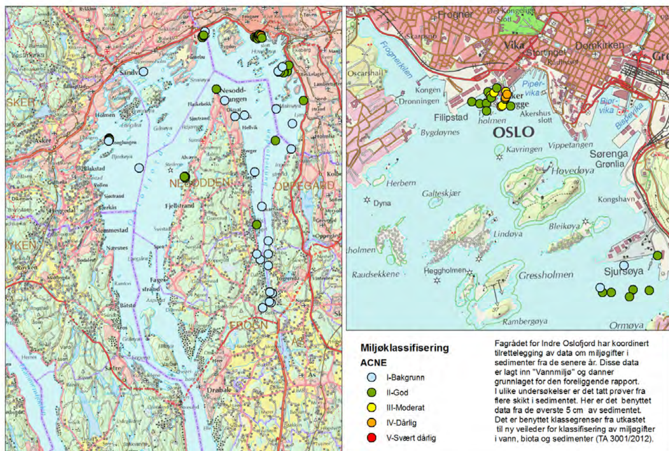
Figur 24. Resultater av klassifisering av miljøtilstand basert på konsentrasjonen av acnaften i de øverste 5 cm av sedimentet i Indre Oslofjord. Klassifiseringen er gjort i henhold til klassegrensene oppgitt i utkast til TA 3001/2012. Venstre side viser resultater for hele Indre Oslofjord. Bildet til høyre viser området nær Oslo i mer detalj. Fargekodene brukt for de enkelte tilstandsklasser er vist i figuren.
