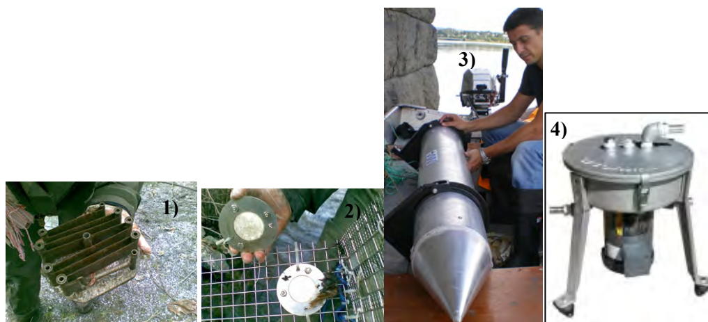
Figur 1. Ulike typer passive prøvetakere av typen 1) SPMD (semipermeable membran device) og 2) POCIS (polar organic chemical integrative sampler), samt høyvolumsprøvetakere 3) sedimentfelle og 4) kontinuerlig vannstrømssentrifuge (vann pumpes fra peristaltisk pumpe til sentrifuge som roterer).
