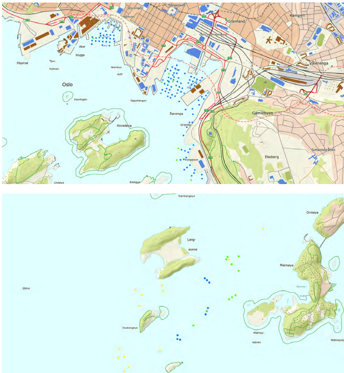
Figur 60. Resultater av klassifisering av miljøtilstand basert på konsentrasjonen arsen i de øverste 0-10 cm av sedimentet i Havneområdet (øverst) og deponiområdet ved Malmøykalven (nederst) i Indre Oslofjord. Resultater som er tatt med i figurene er data som forelå pr 06.09. 2013 fra alle prøver tatt etter 01.01.2009. Klassifiseringen er gjort i henhold til klassegrensene oppgitt i utkast til TA 3001/2012. Fargekodene brukt for de enkelte tilstandsklasser er vist i Figur 55 . Kilde: Figurer tilsendt fra Plan, utbygging og miljø/Miljø, Oslo Havn KF
