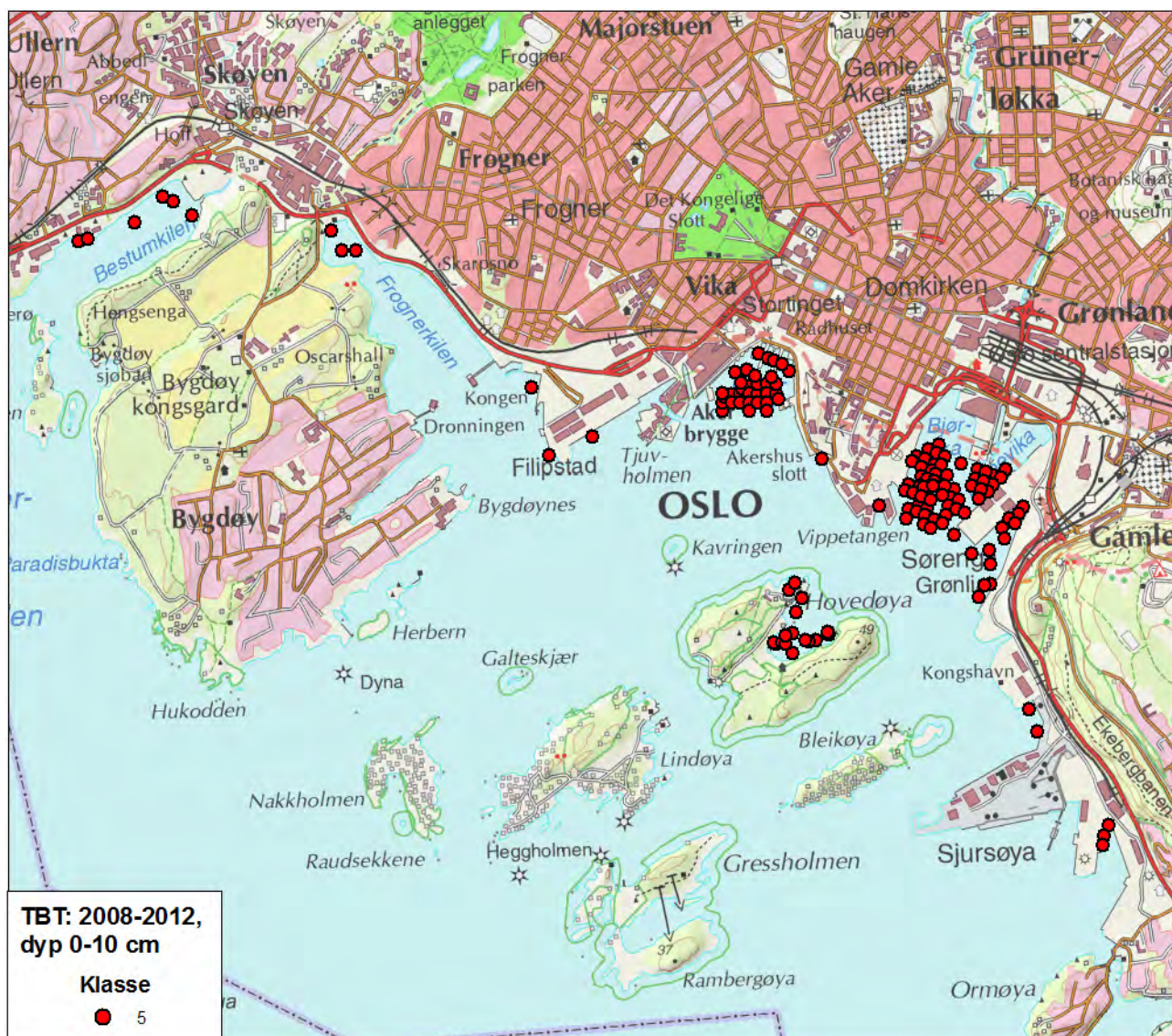
Figur 75. Resultater av klassifisering av miljøtilstand basert på konsentrasjonen av tributyltinn (som kation) i de øverste 0-10 cm av sedimentet i Indre Oslofjord, prøver tatt i perioden 2008-2012. Klassifiseringen er gjort i henhold til klassegrensene oppgitt i utkast til TA 3001/2012. Fargekodene brukt for de enkelte tilstandsklasser er vist i figuren.
